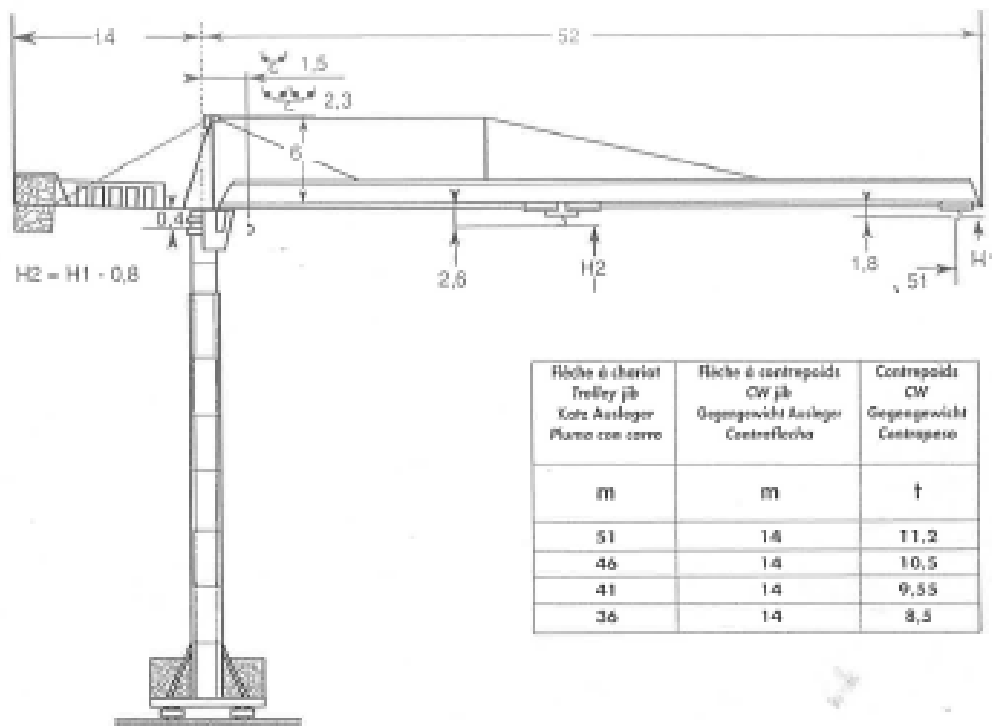
FLECHE - JIB - AUSLEGER - FLECHA 51 m
